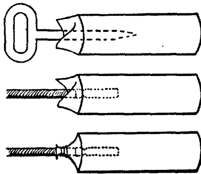
Fig 1 DYNAMITE PRIMER
